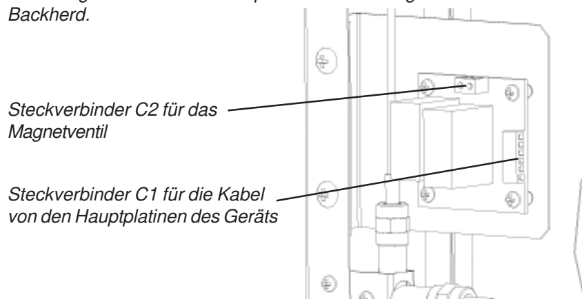
Abbildung 4: Einbau der Relaisplatine und des Magnetventils am Backherd.
