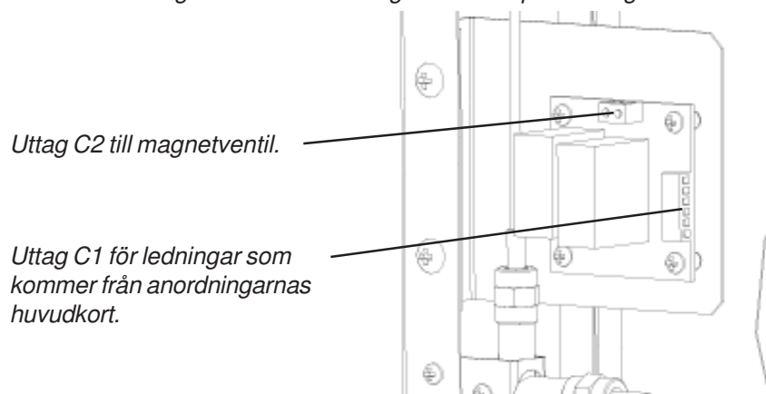
Bild 4: Montering av reläkort och magnetventil i spis med ugn.
